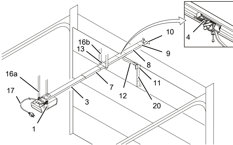
Afb. 1: Productoverzicht
