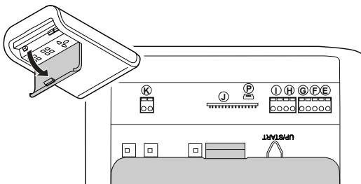
Afb. 7: Afdekking van de aandrijfkop openen
