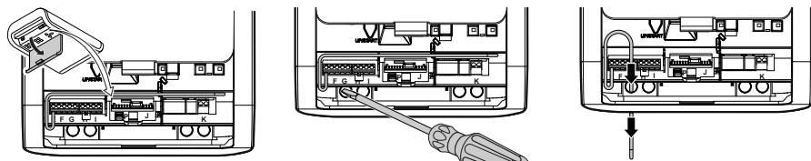
Afb. 8: Antenne leggen
